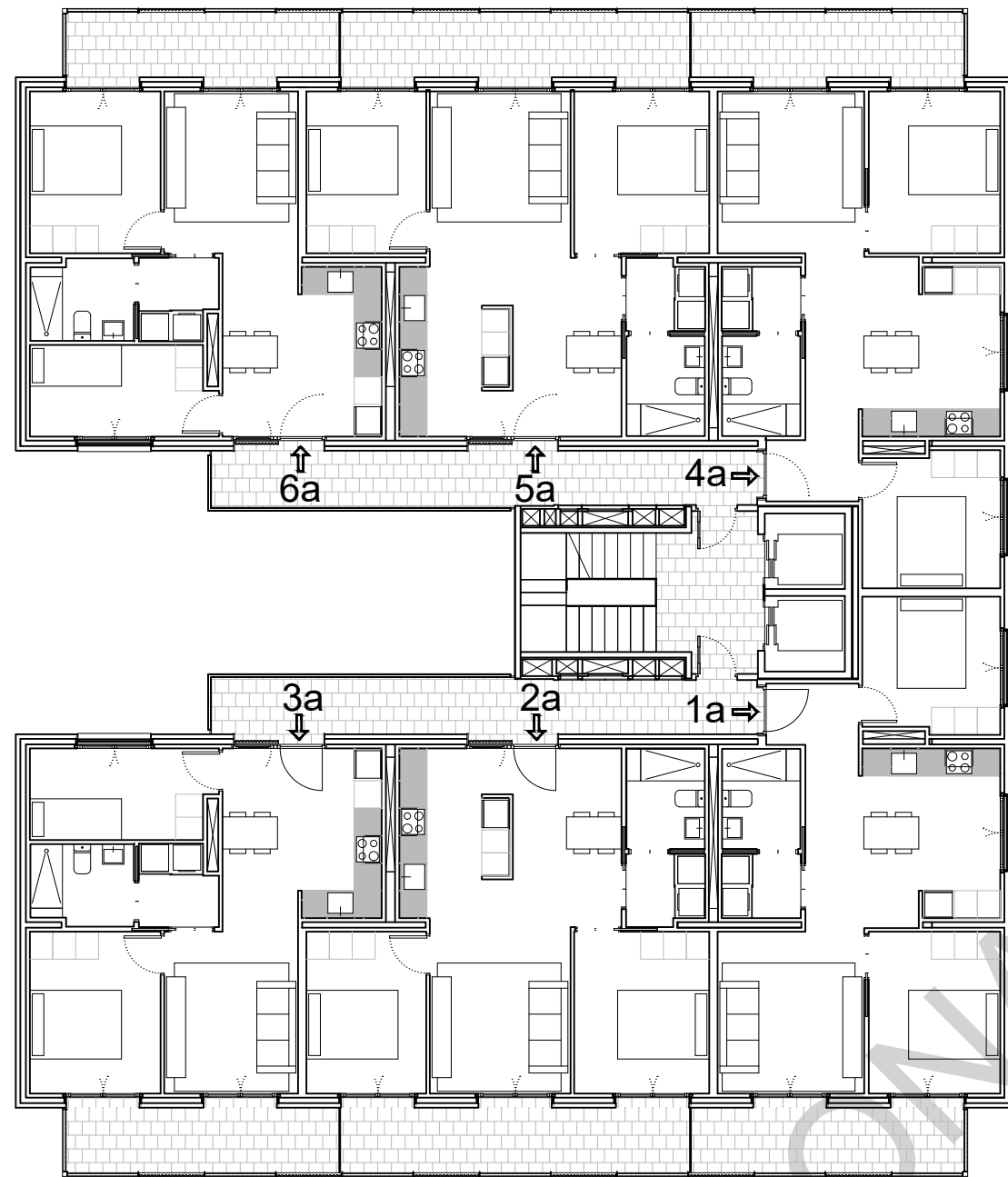
PLANTA CINQUENA
