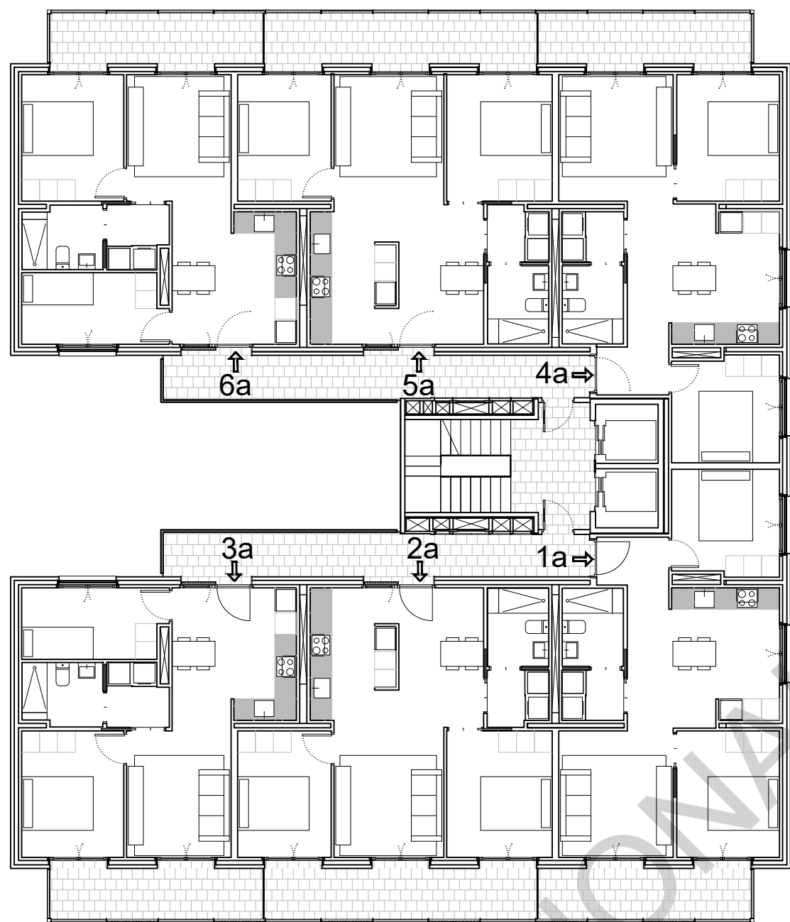
PLANTA TERCERA
