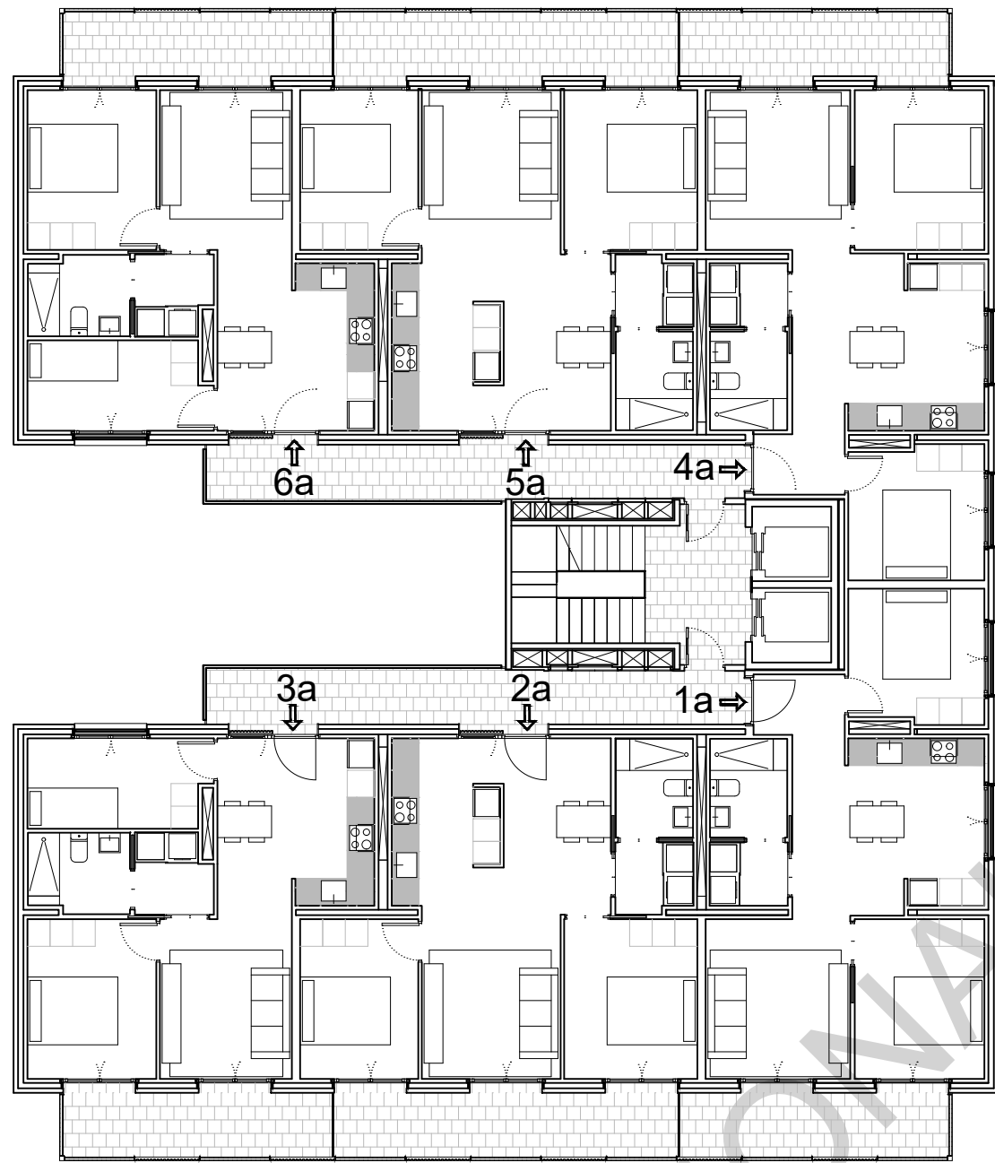
PLANTA SETENA
