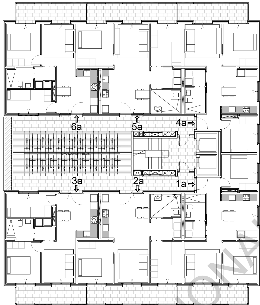
PLANTA PRIMERA
