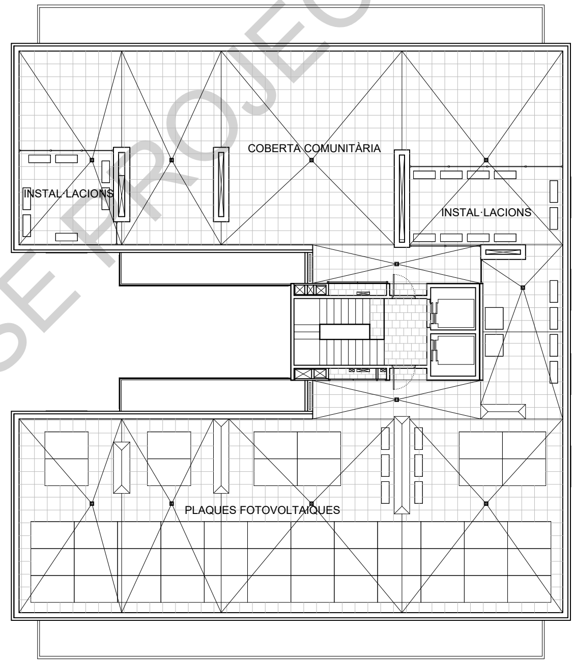
PLANTA COBERTA
