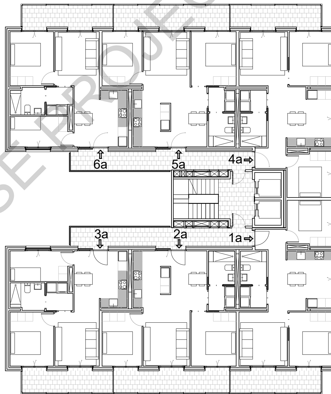
PLANTA QUARTA
